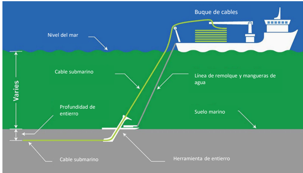
Esquema del proceso de instalación de un cable
